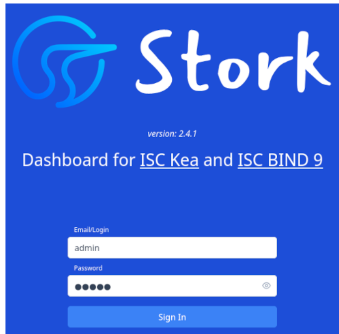
Figura 7: Interfície web
